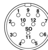
Polbild Buchsenstecker mit Außengewinde 17-polig Ansicht auf Steckseite
