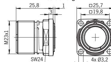
Maßzeichnung
